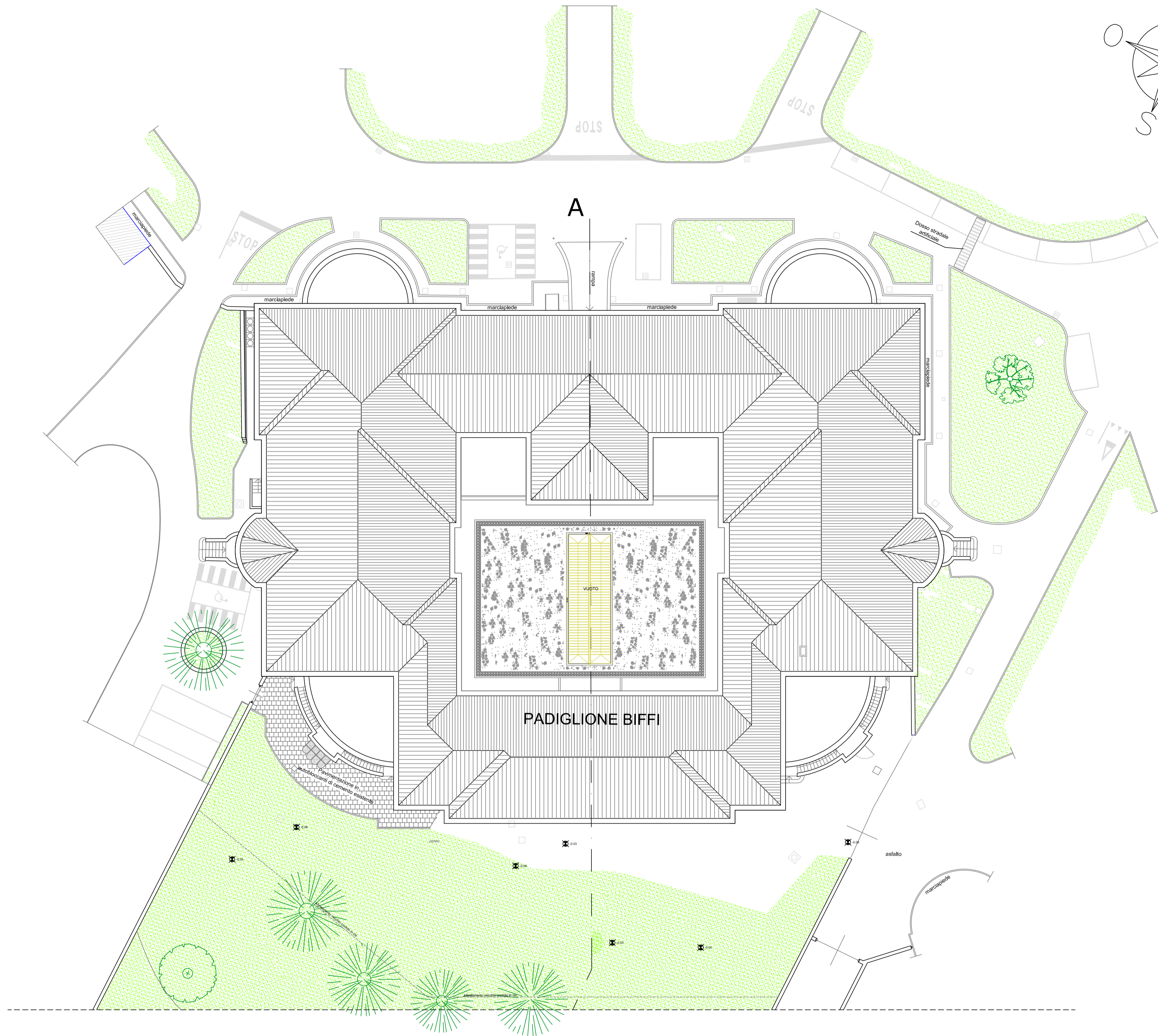
Planimetria generale Stato di fatto Scala 1:200
